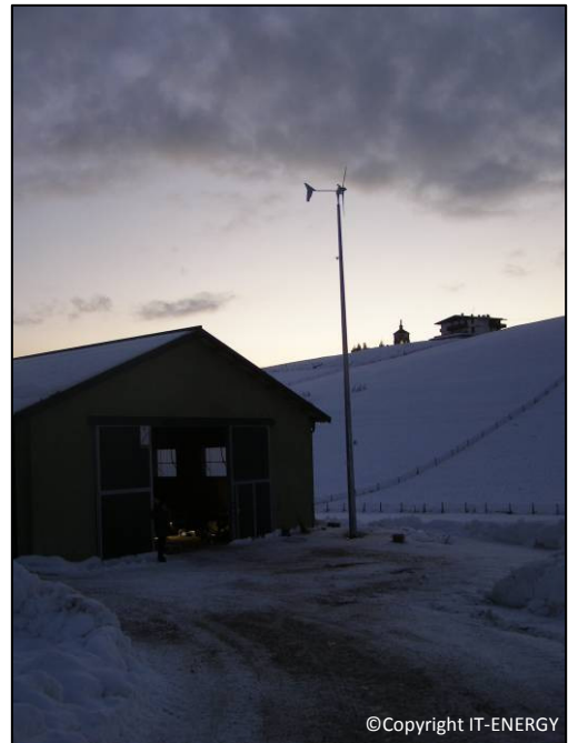
Impianto in isola realizzato a Gallio (VI)
